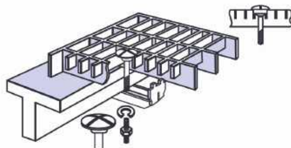
КРЕПЛЕНИЕ ПРЕССОВАННОГО НАСТИЛА С МАЛОЙ ЯЧЕЙКОЙ
